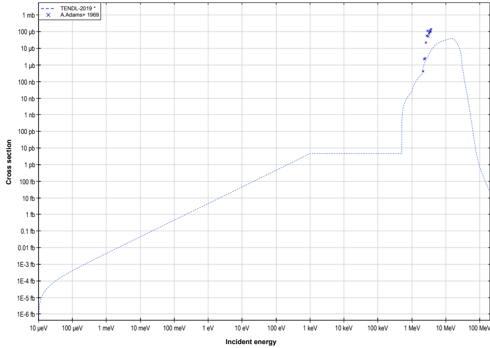
O18 ( \alpha,\gamma ) or Ne22 production log-log
