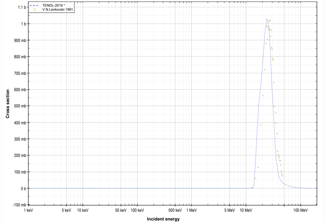
Ge73 ( \alpha, 2n ) or Se75 production lin-log
