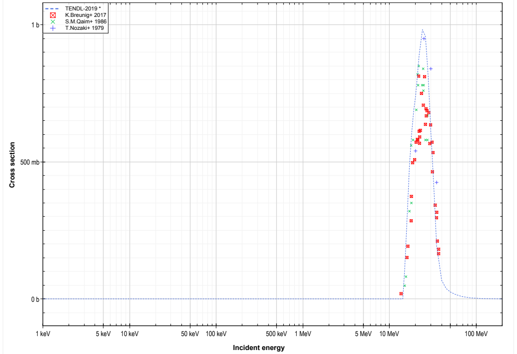
As75 ( \alpha, 2n ) or Br77 production lin-log
