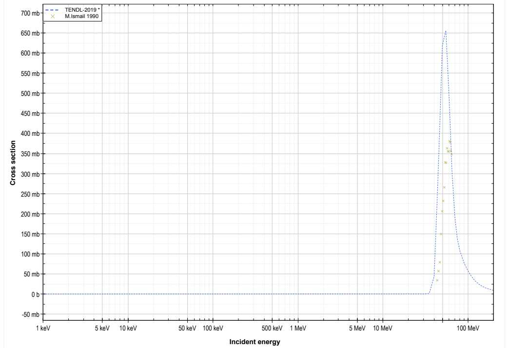
Ga69 ( \alpha, n+t ) or Ge69 production lin-log
