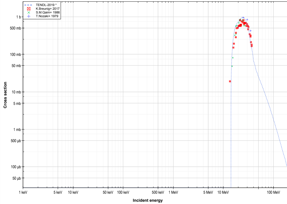
As75 ( \alpha, 2n ) or Br77 production log-log
