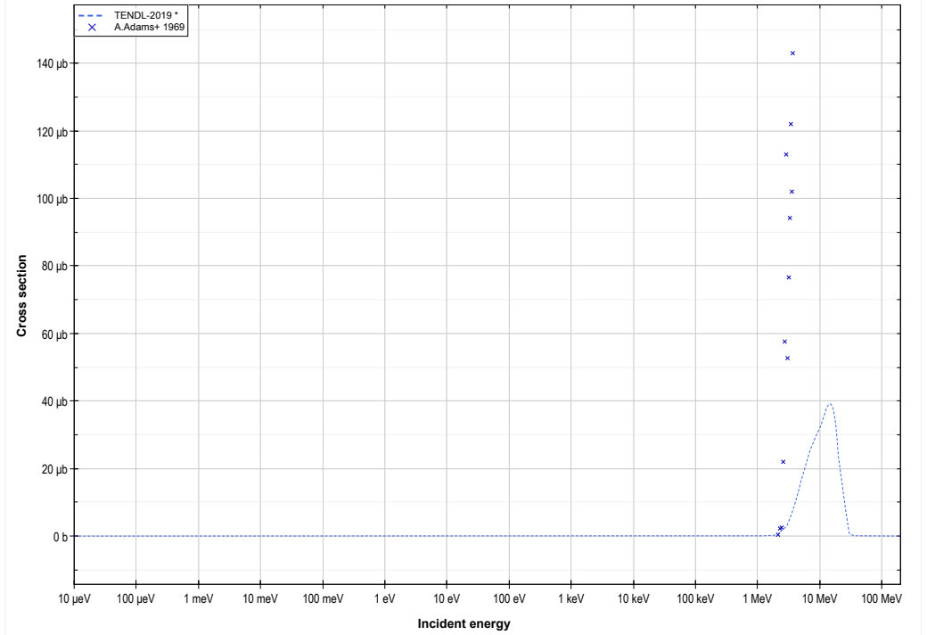
O18 ( \alpha,\gamma ) or Ne22 production lin-log
