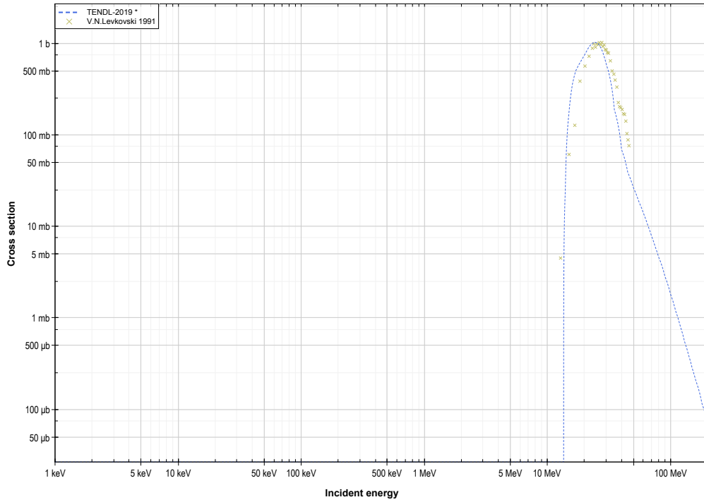
Ge73 ( \alpha, 2n ) or Se75 production log-log
