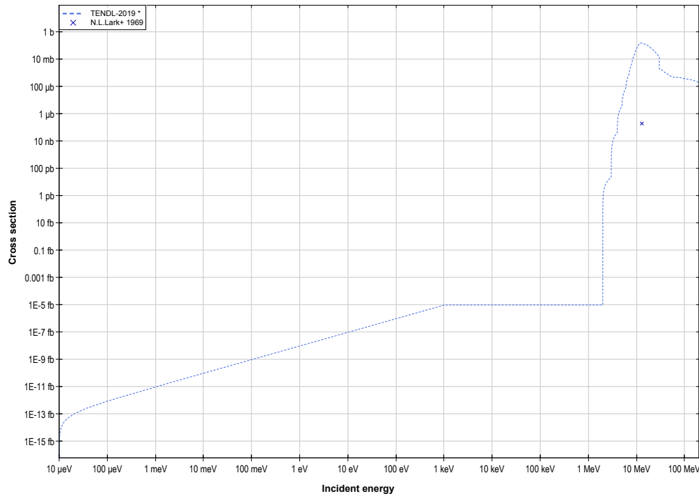
U234 (d,p) or U235 production log-log
