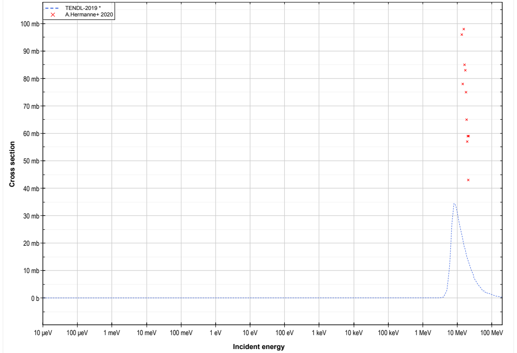
Te130 (d,n) or I131 production lin-log
