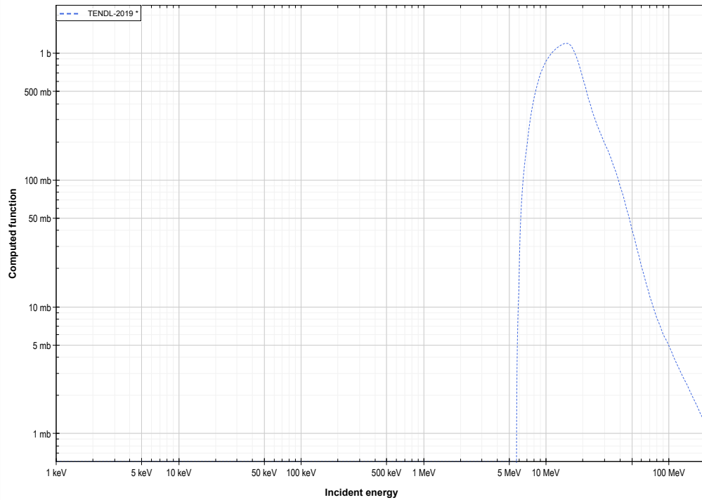
Ge74 (d,2n) or As74 production log-log
