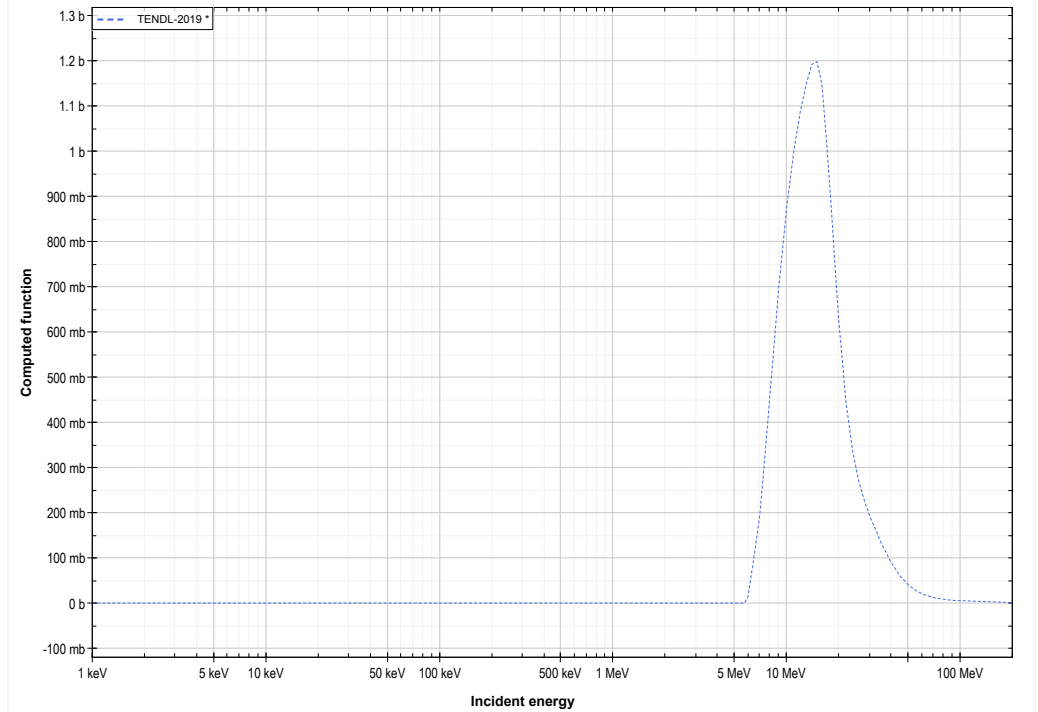
Ge74 (d,2n) or As74 production lin-log
