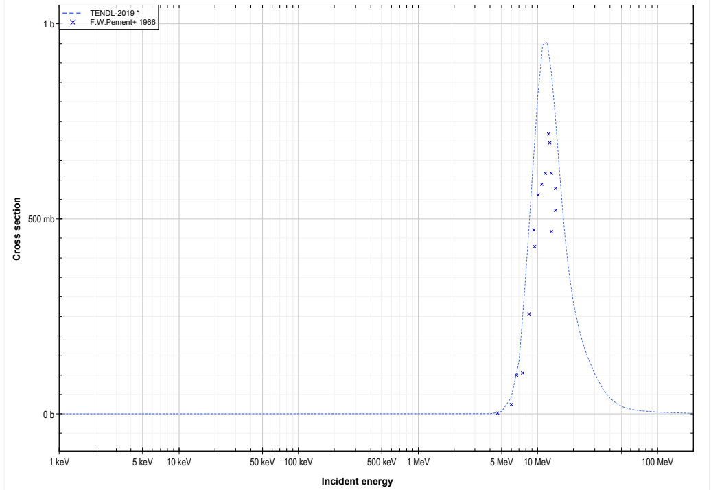
Te130 (d,2n) or I130 production lin-log
