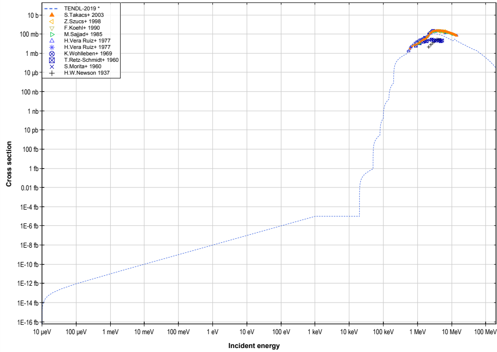
N14 (d,n) or O15 production log-log
