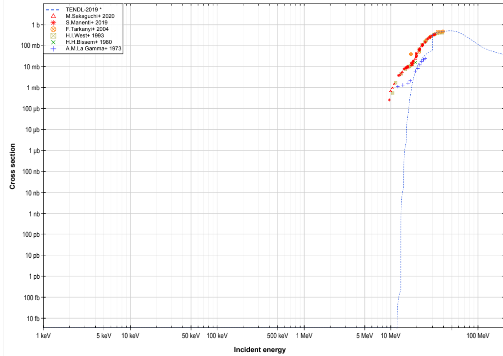
Y89 (d,n+d) or Y88 production log-log
