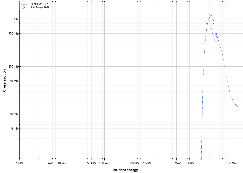
Tl205 (d,4n) or Pb203 production log-log
