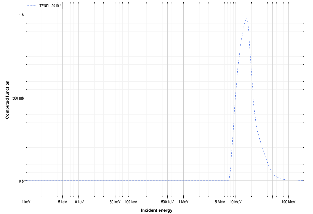
Mo94 (d,2n) or Tc94 production lin-log
