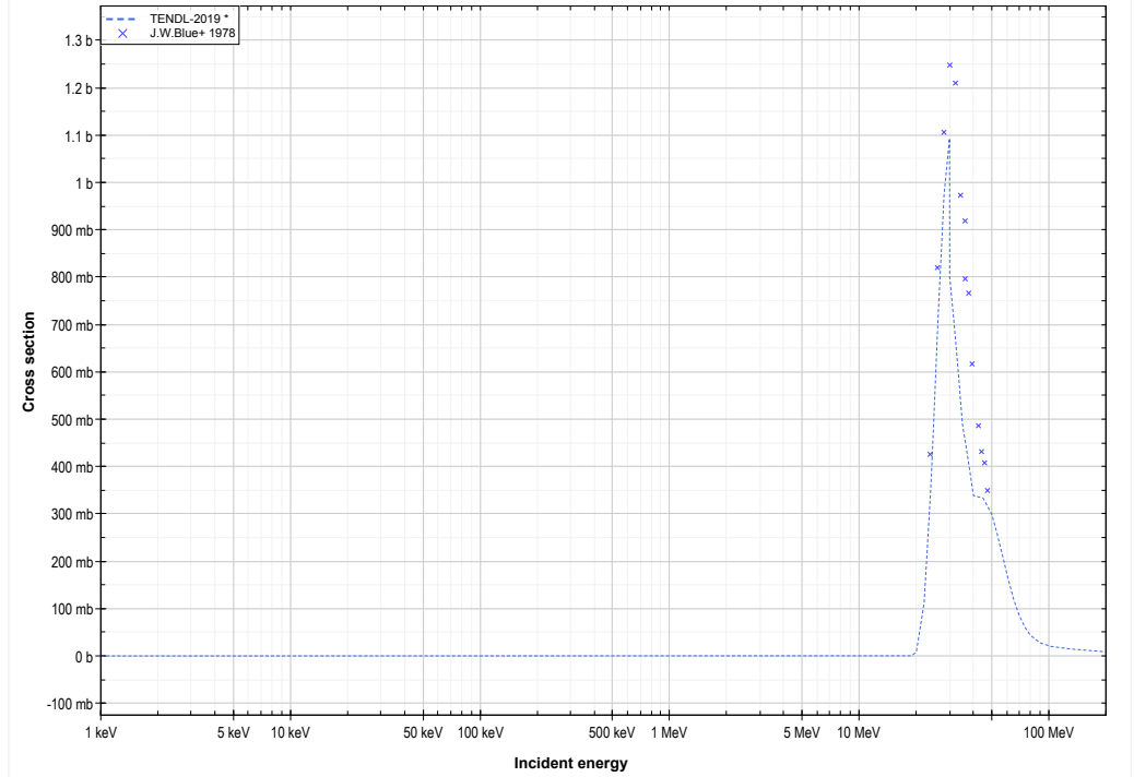
Tl205 (d,4n) or Pb203 production lin-log
