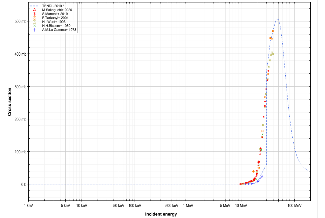
Y89 (d,n+d) or Y88 production lin-log
