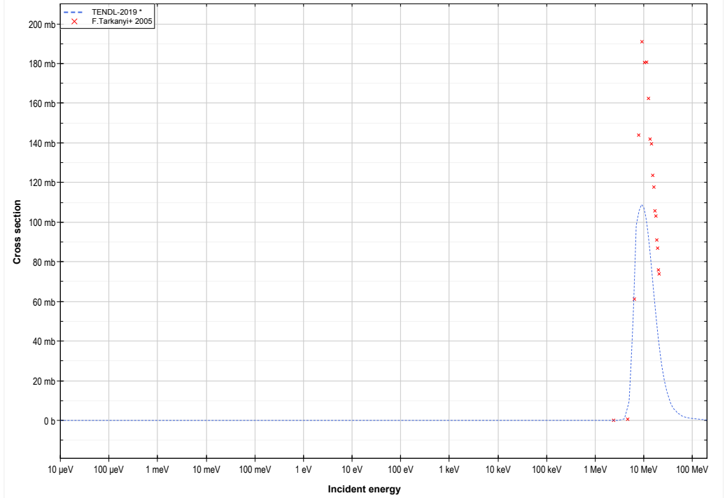
Cd114 (d,p) or Cd115 production lin-log
