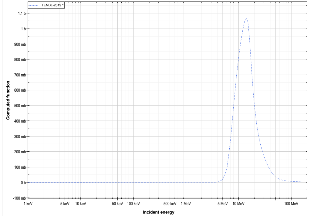
Nb93 (d,2n) or Mo93 production lin-log
