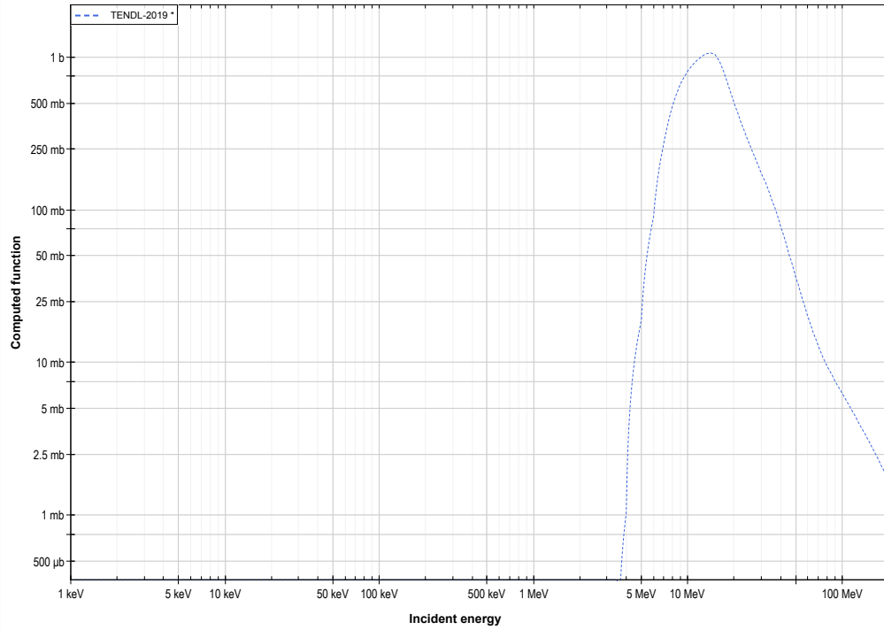
Nb93 (d,2n) or Mo93 production log-log
