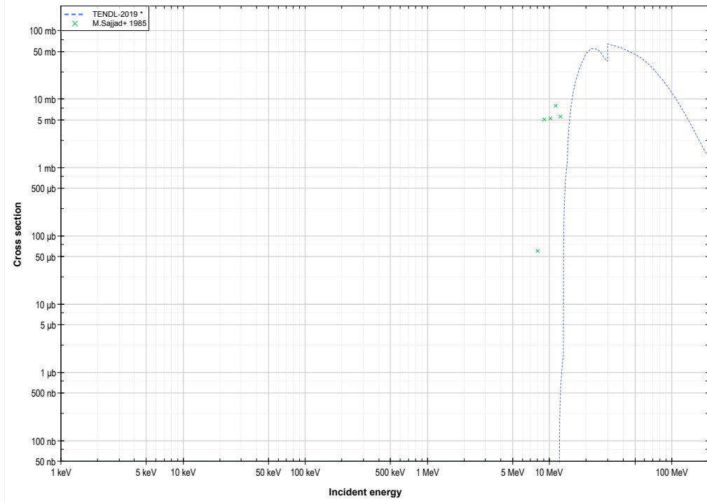
N14 (d,n+d) or N13 production log-log
