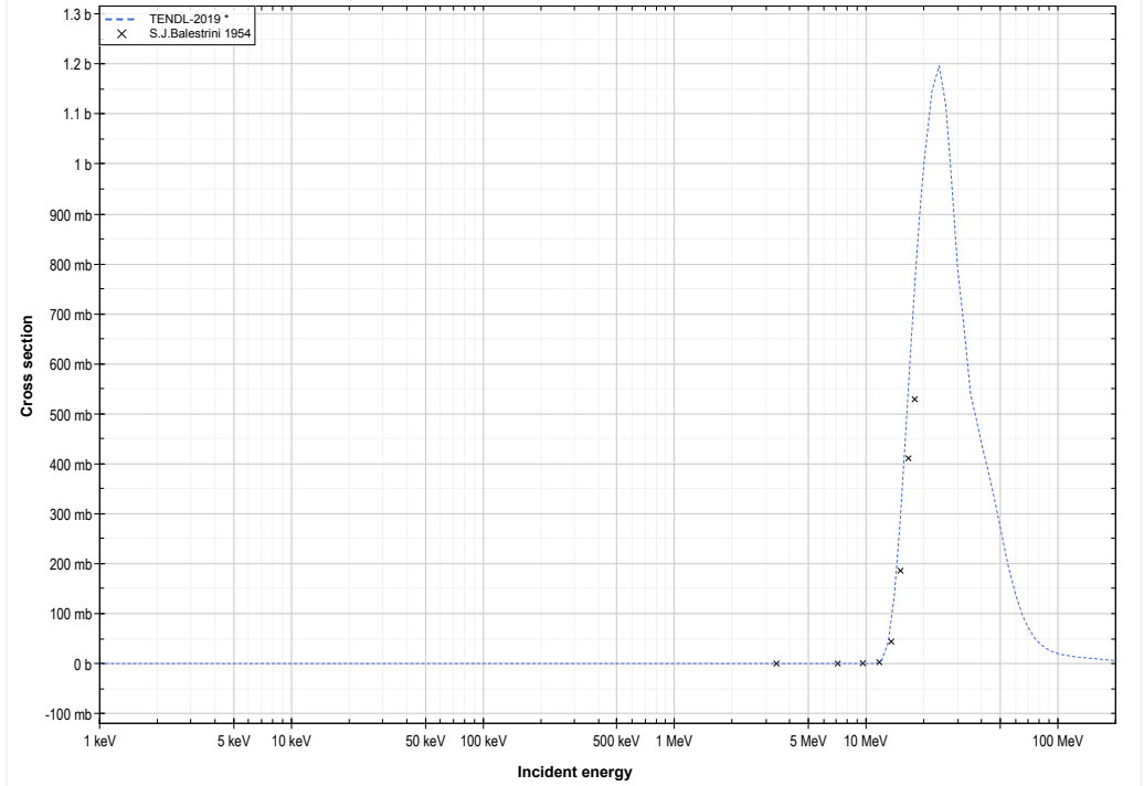
I127 (d,3n) or Xe126 production lin-log
