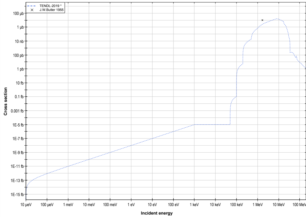
O16 (d, \gamma ) or F18 production log-log
