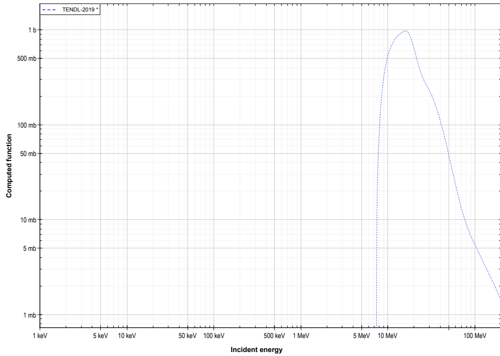
Mo94 (d,2n) or Tc94 production log-log
