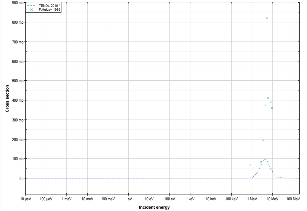
Ne22 (d,p) or Ne23 production lin-log
