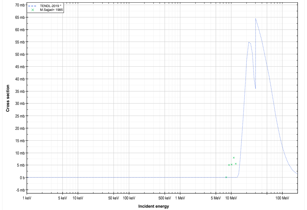
N14 (d,n+d) or N13 production lin-log
