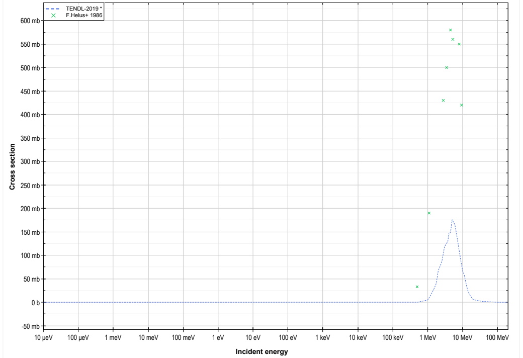
Ne20 (d,n) or Na21 production lin-log
