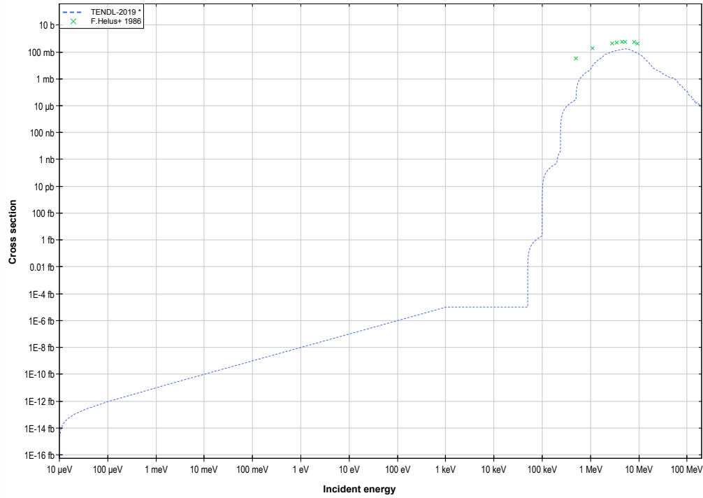
Ne20 (d,n) or Na21 production log-log
