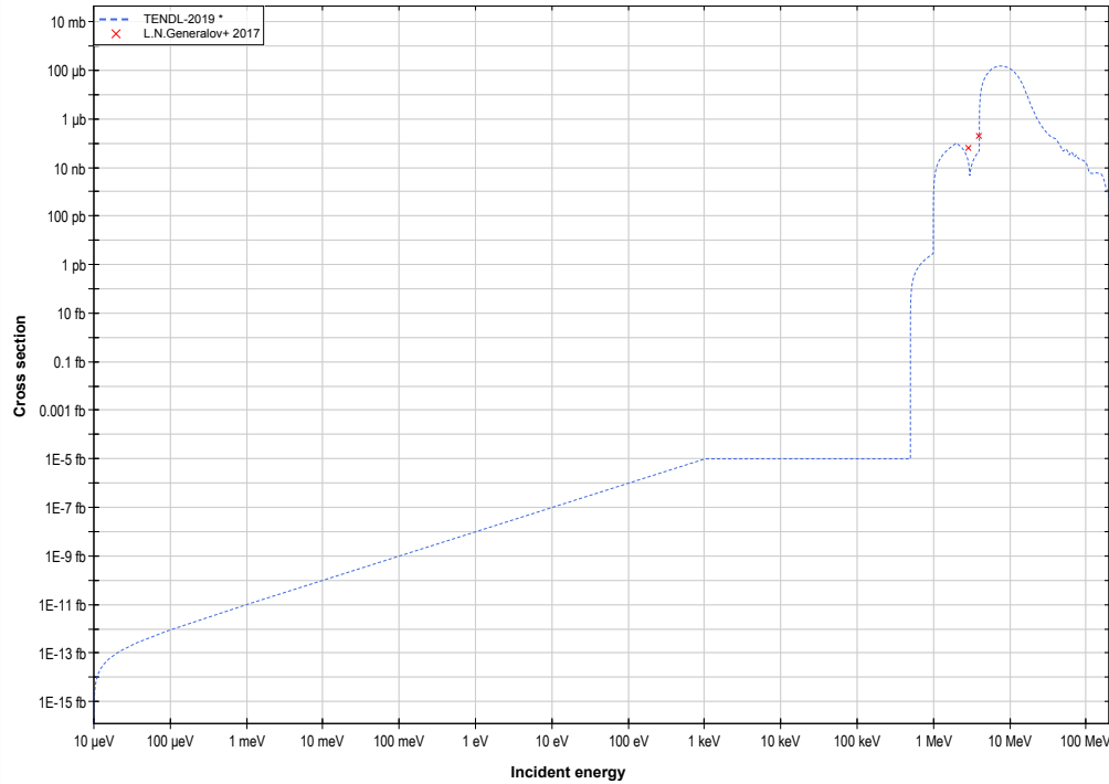
Cu63 (d, \gamma ) or Zn65 production log-log
