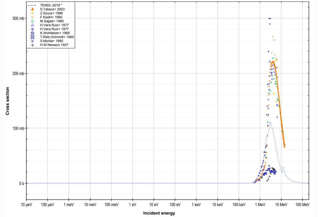
N14 (d,n) or O15 production lin-log
