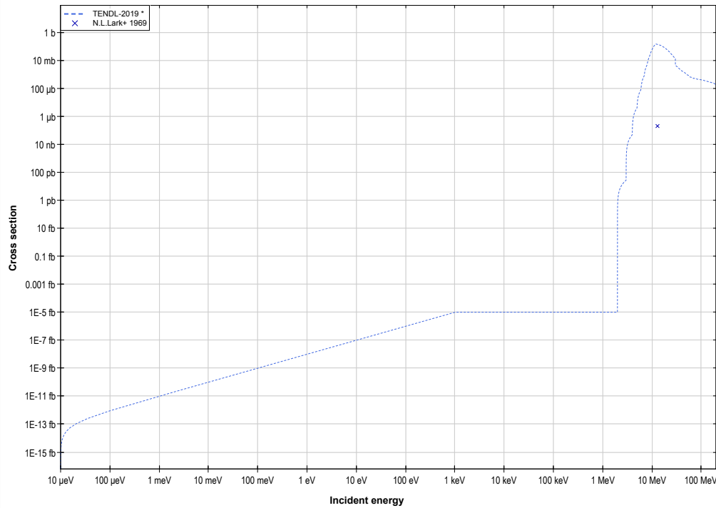
U236 (d,p) or U237 production log-log
