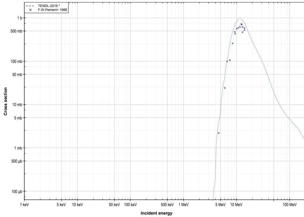
Te130 (d,2n) or I130 production log-log
