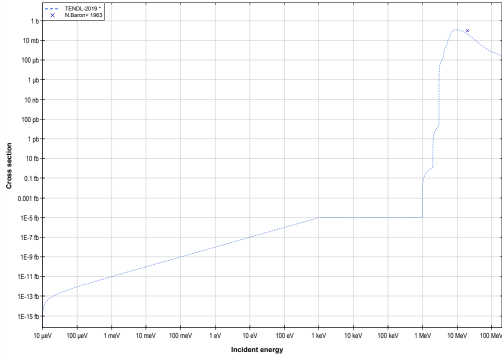
Ba138 (d,p) or Ba139 production log-log
