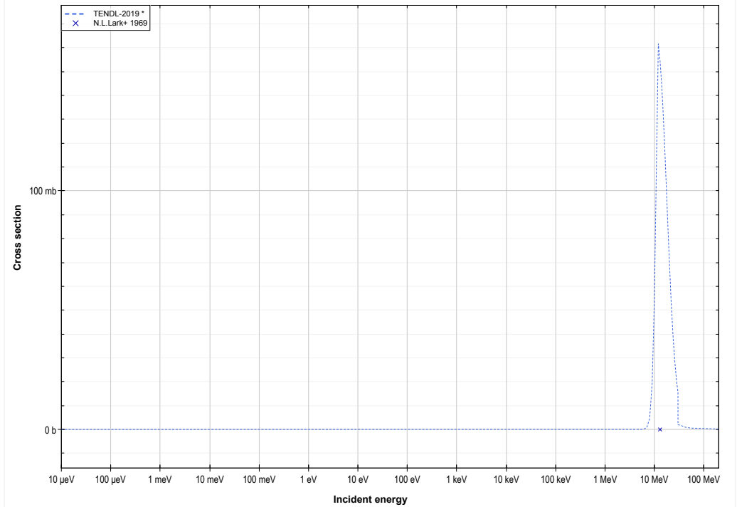
U234 (d,p) or U235 production lin-log
