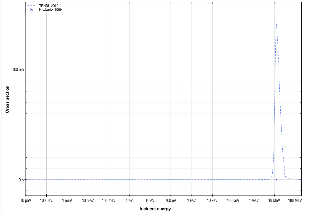
U236 (d,p) or U237 production lin-log
