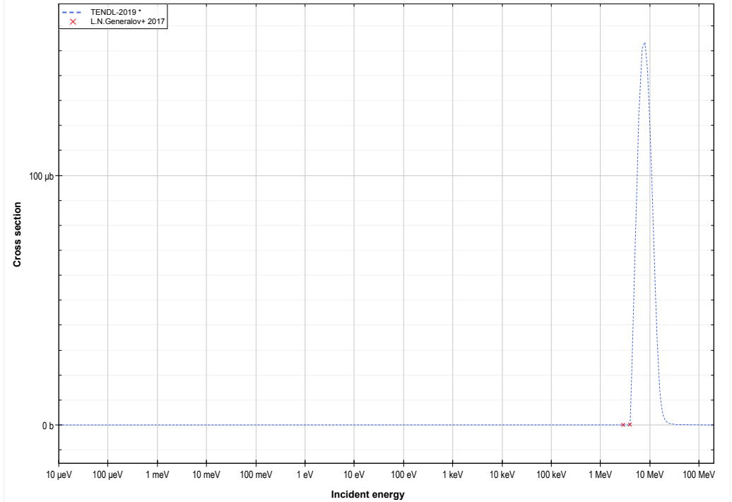
Cu63 (d, \gamma ) or Zn65 production lin-log
