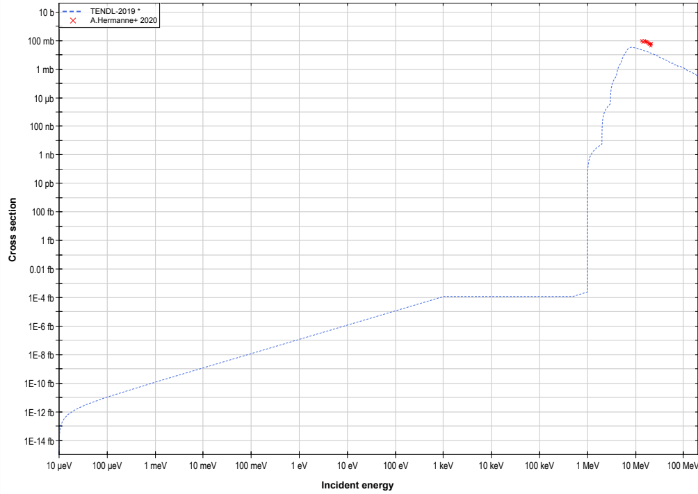
Te130 (d,n) or I131 production log-log
