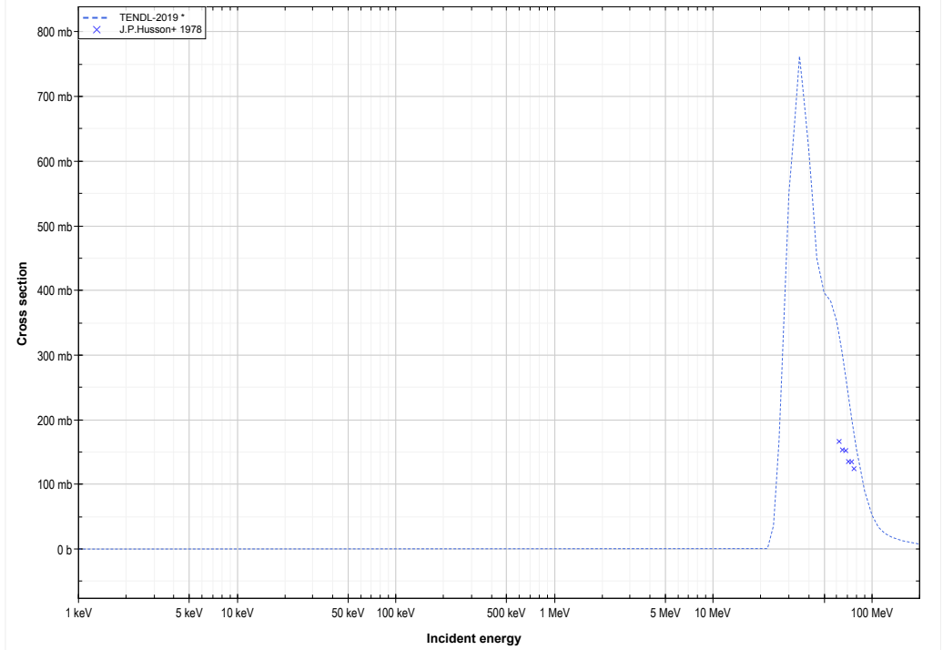
I127 (d,4n) or Xe125 production lin-log
