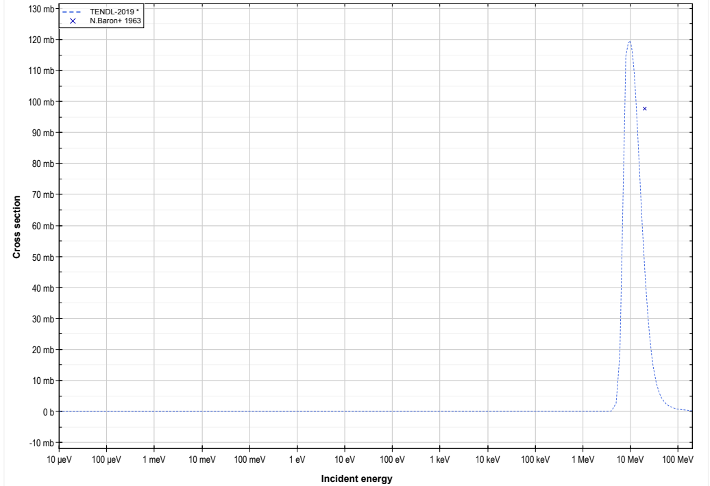
Ba138 (d,p) or Ba139 production lin-log
