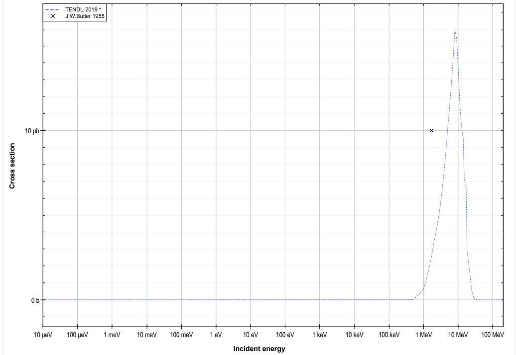
O16 (d, \gamma ) or F18 production lin-log
