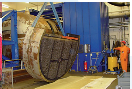
在暫時儲存設施 (Interim Storage Facility North, ZLN) 利用大帶鋸切割蒸氣產生器
