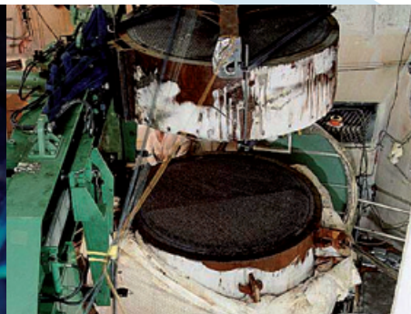
用冰鋸技術拆除蒸氣產生器
