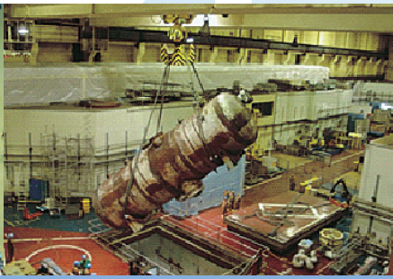
拆除 4 號機的一具蒸氣產生器
