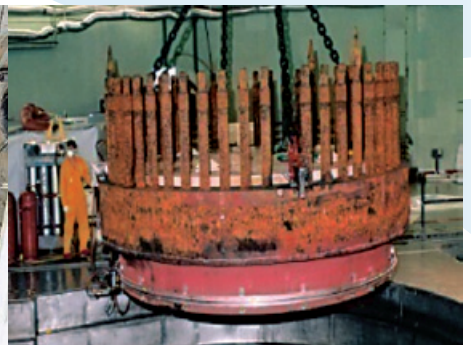
拆除反應爐壓力容器 - 吊移 Flange
